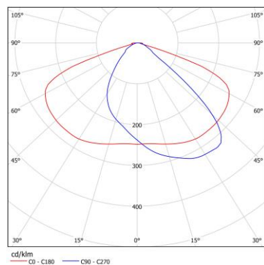
Рисунок 3 Типы КСС
